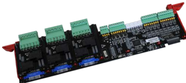
EDG-P-8I-6R-4V-P
