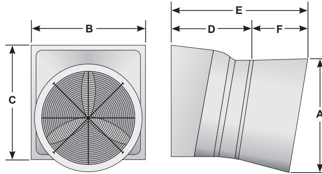
Fan Dimensions
